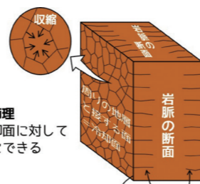
柱状節理…冷却面に対して垂直にできる 岩脈の縁 冷却面に対して垂直にできた割れ目
